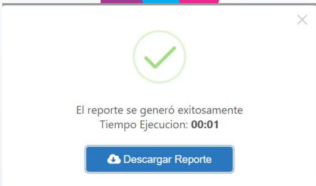
Figura 12 - Descarga reporte
