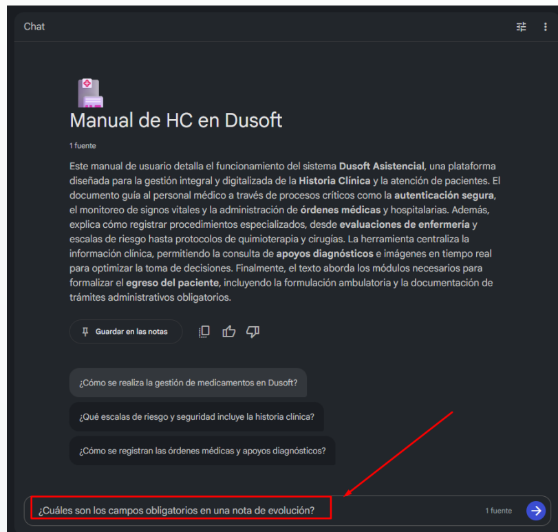
Figura 2 - Consulta inteligente
