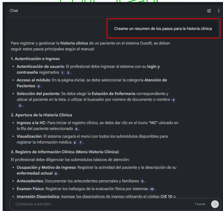
Figura 6 - Resumen
